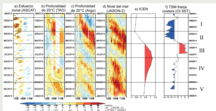
Figura 1. Evolución durante el año 2014 de las anomalías del a) esfuerzo de viento zonal, b-c) profundidad de la isoterma de 20°C, y d) nivel del mar a lo largo de la línea ecuatorial, así como del e) Índice Costero El Niño y f) temperatura superficial del mar a 25-50 km de la costa entre 13° S y 5° S (en rojo se indican valores > 0.4 y en azul < -1). Las fases descritas en el texto se indican a la derecha.
