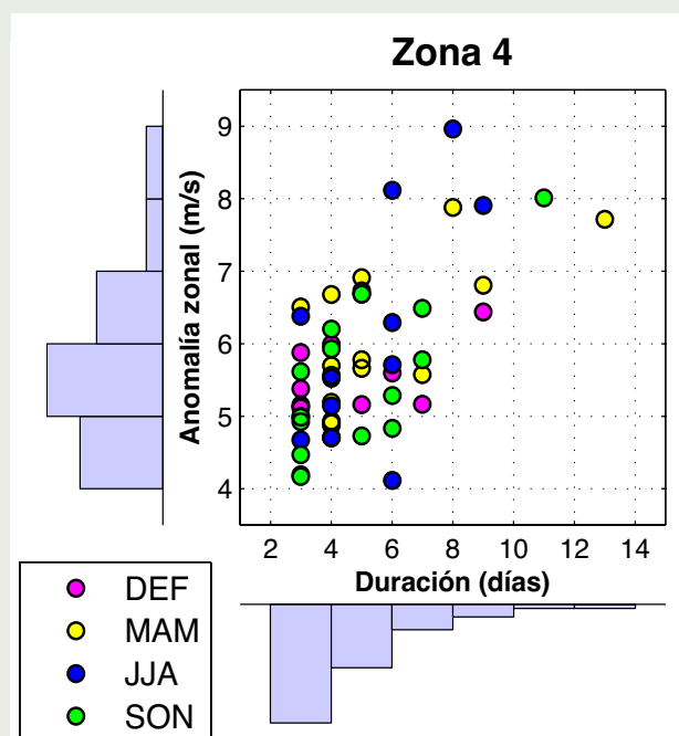
Figura 2. Dispersión entre la duración y la anomalía de viento zonal máxima de cada evento en Z4. Los colores indican diferentes estaciones del año.
