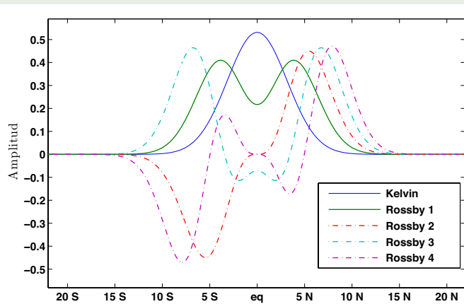
Figura 1. Estructuras meridionales para el nivel del mar del modo Kelvin y los cuatro primeros modos Rossby.
