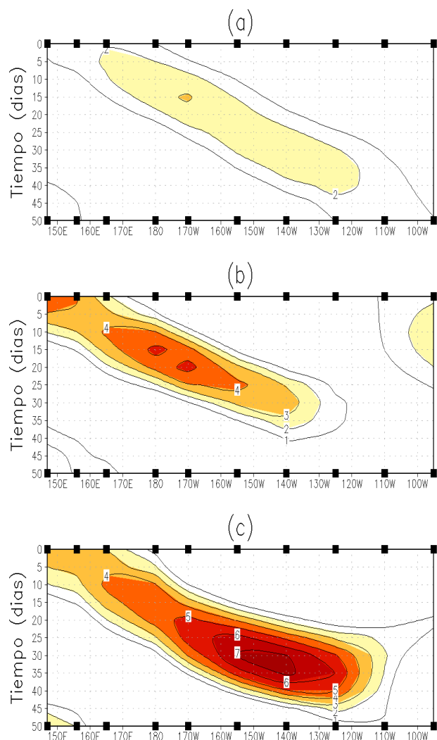
Figura 1. Promedio de los patrones de evolución de la anomalía intraestacional de la profundidad de la isoterma de 20°C (termoclina) en metros a lo largo de la franja ecuatorial relacionado a un forzante de viento intraestacional de (a) entre 3 y 4 m/s, (b) 4 y 5 m/s y (c) vientos mayores a 5 m/s. Los cuadrados a lo largo de los ejes superior e inferior indican la posición de las boyas del proyecto TAO.
